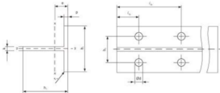
Soğuk çekme düz bağı ve kanat flanşlı kılavuz ray
